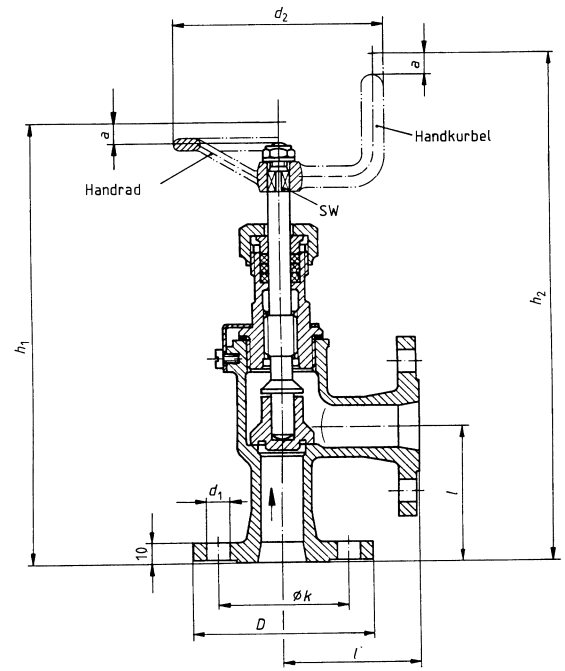
Form D Rückschlag-Eckventil, metallisch dichtend
