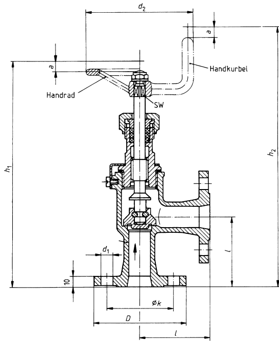
Form B Absperr-Eckventil, metallisch dichtend
